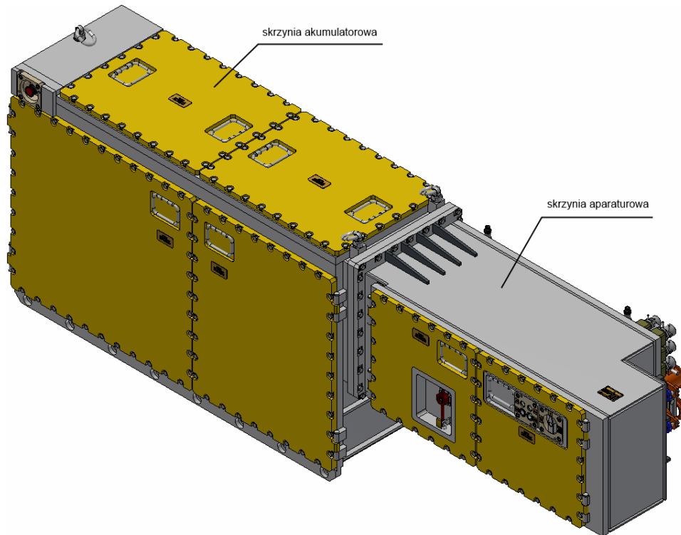
Rys. 1. Model przestrzenny zespołu zasilająco-sterującego HK-1 spągokoladarki [14]
