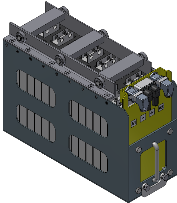
Rys. 6. Kompletny szufladowy moduł baterijny [14]
