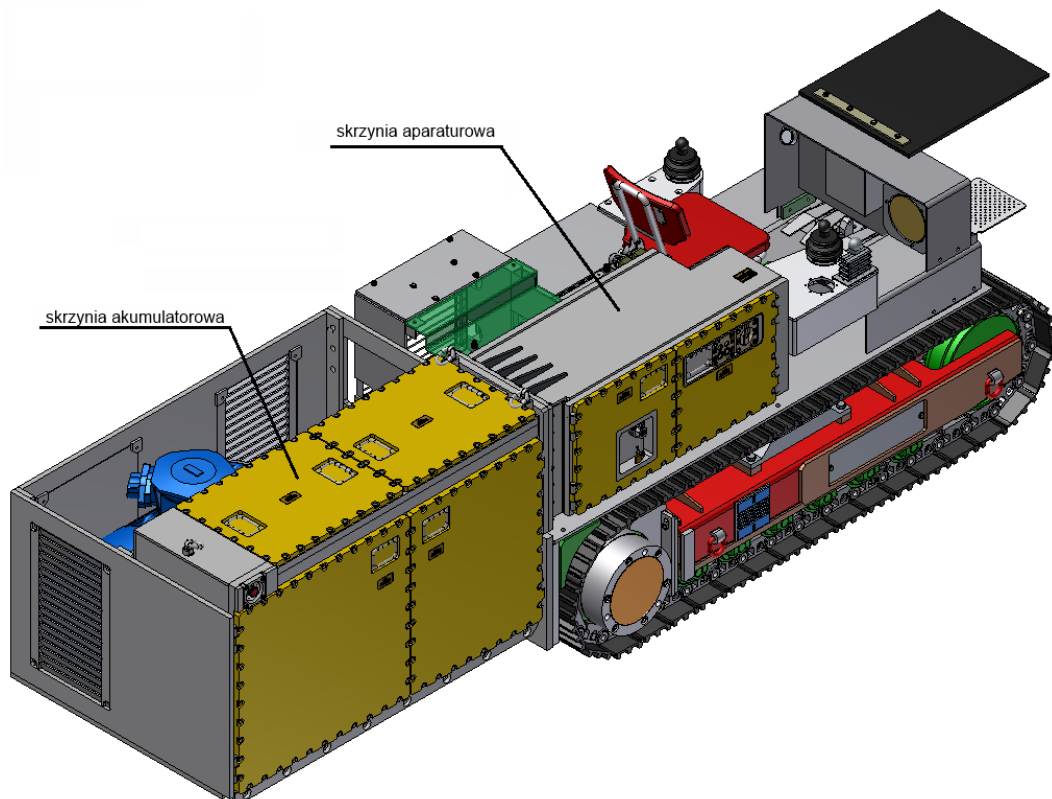
Rys. 2. Sposób zabudowy zespołu zasilająco-sterującego HK-1 na podwoziu spągokoladarki [14]
