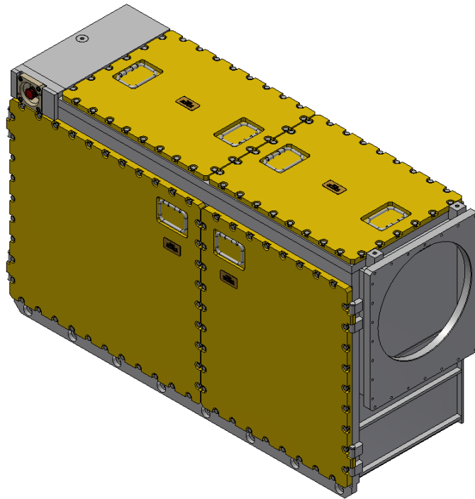
Rys. 3. Skrzynia akumulatorowa [14]
